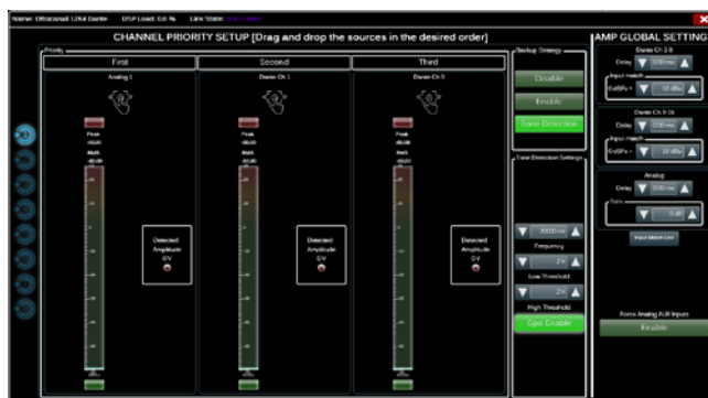
Рис. 4: Ottocanali DSP+D: выбор входа и правила резервирования
